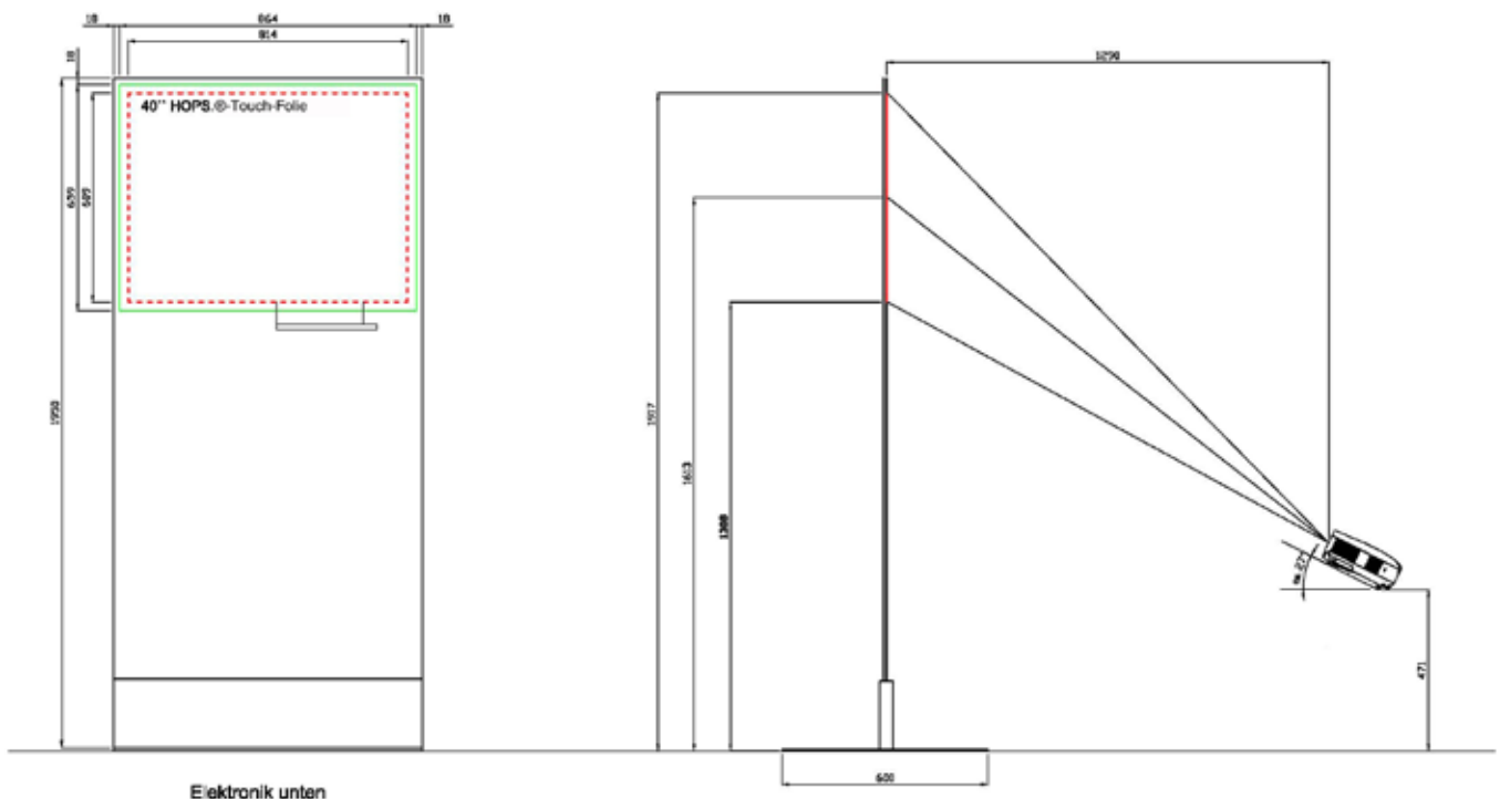
Beispiel einer HOPS.®-Ancora-Touch 40" mit 38° Projektionswinkel
